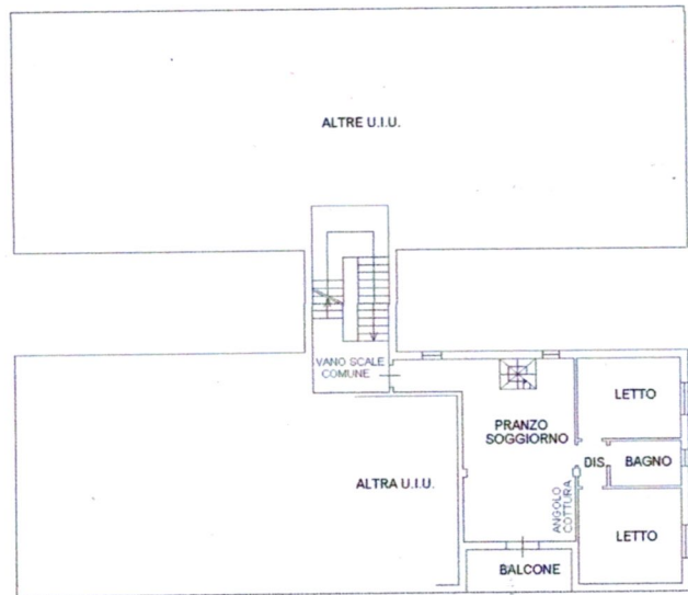
PIANO SECONDO H 2.70
